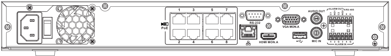
DIVAR network 2000 (8 PoE) 後方面板
