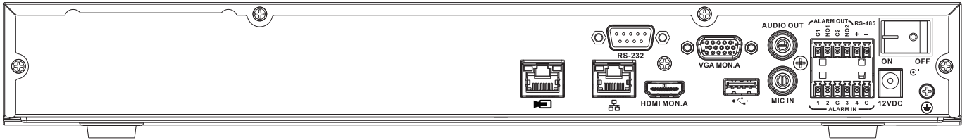
DIVAR network 2000 (無 PoE) 後方面板
