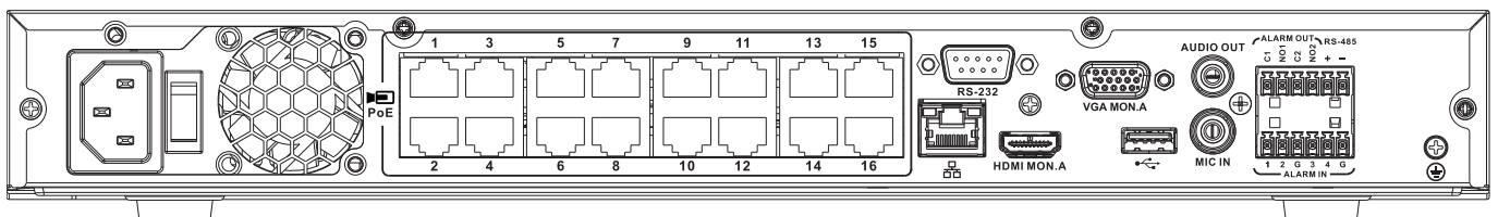
DIVAR2000 网络 (16 PoE) 后面板
