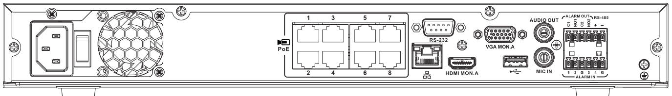
DIVAR2000 网络 (8 PoE) 后面板
