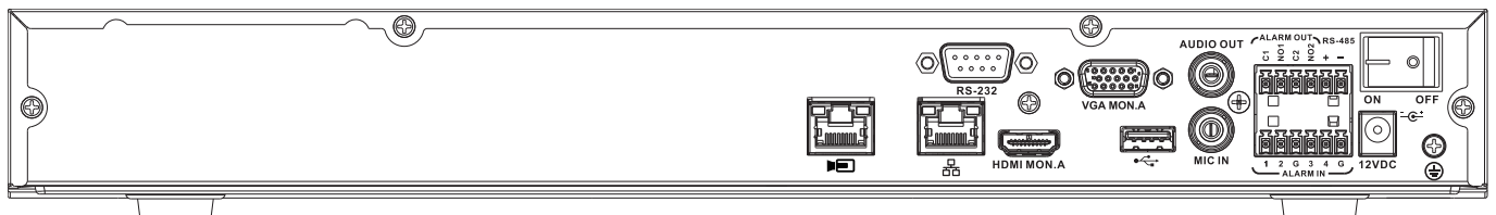
DIVAR2000 网络 (无 PoE) 后面板
