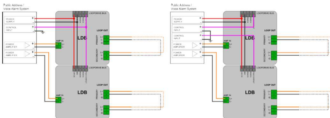
Afbeelding 4.3: Bedrading met meerdere LDB's. Links: afzonderlijke stringscontactingangen. Rechts: gemeenschappelijk stringcontact
