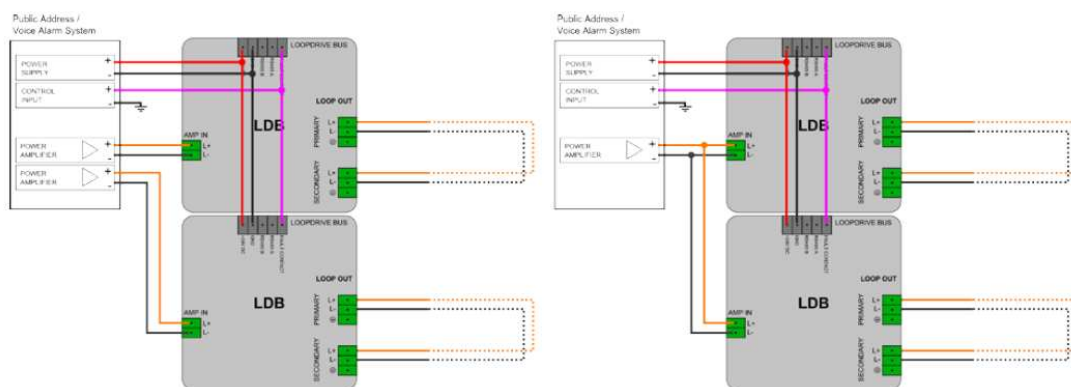
Afbeelding 4.2: Bedrading met meerdere LDB's. Links: afzonderlijke versterkerkanalen. Rechts: gedeelde versterker
