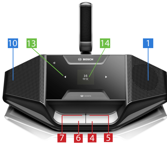
Şekil 3.4: DCNM-DSL
