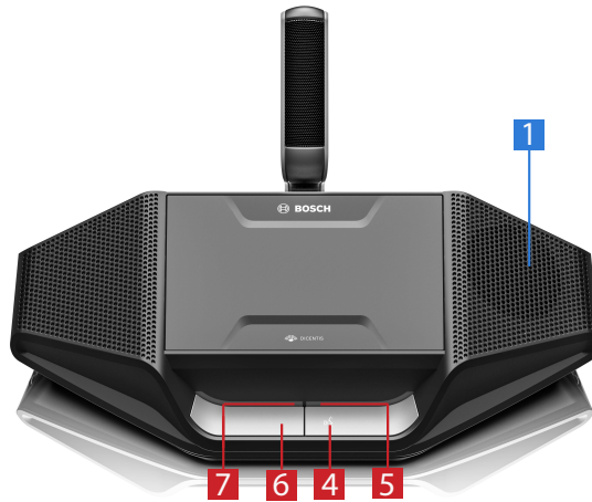
Şekil 3.2: DCNM-D
