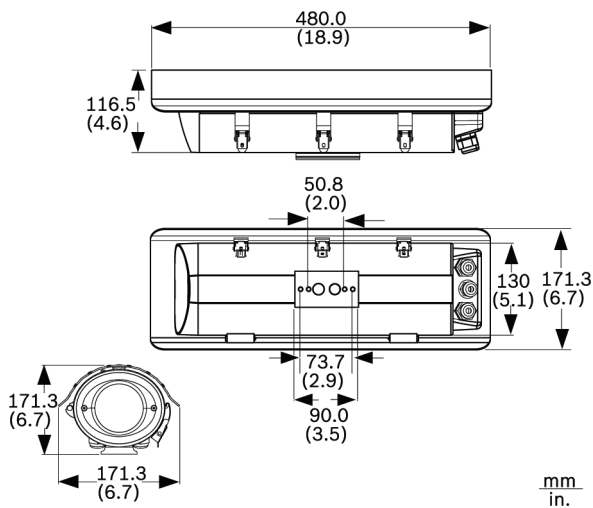
Размеры в мм для внутренних кожухов UHI-OG(S)-0
