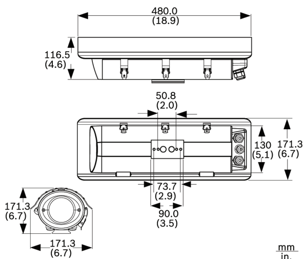
Dimensões em mm para caixas para interior UHI-OG(S)-0
