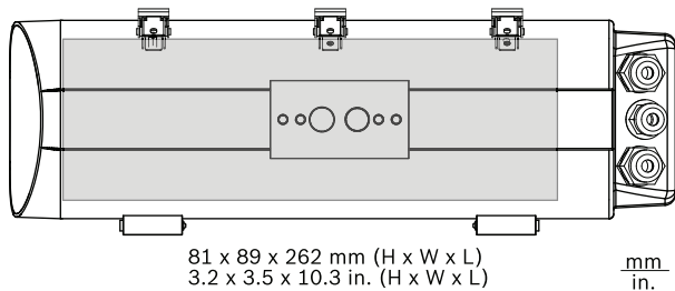
Dimensões em mm, espaço interior máximo utilizável (baseado no tamanho da câmara/objectiva)
