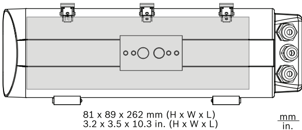
Afmetingen in mm voor alle uitvoeringen, maximaal beschikbare interne ruimte (gebaseerd op afmetingen van camera en objectief)
