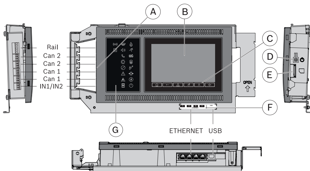
Přehled řídicí jednotky ústředny
