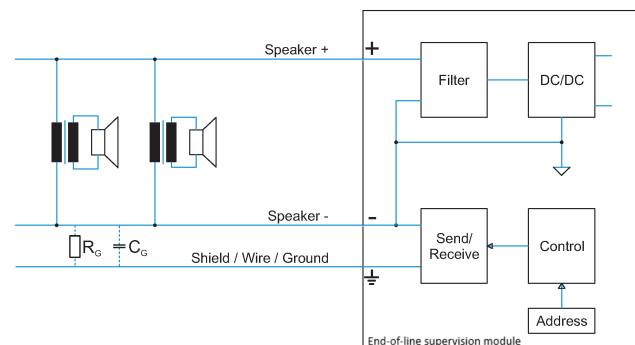
Diagrama do circuito
