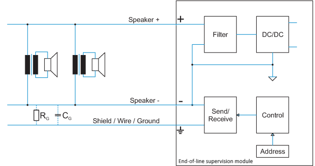
Kytentäkaavio
