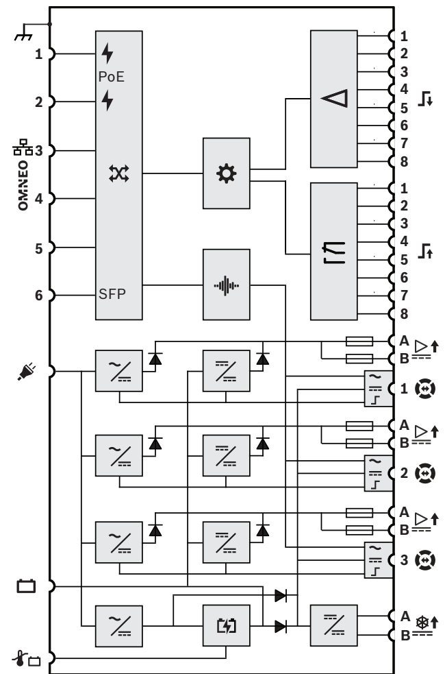
Diagrama funcional e de conexão
