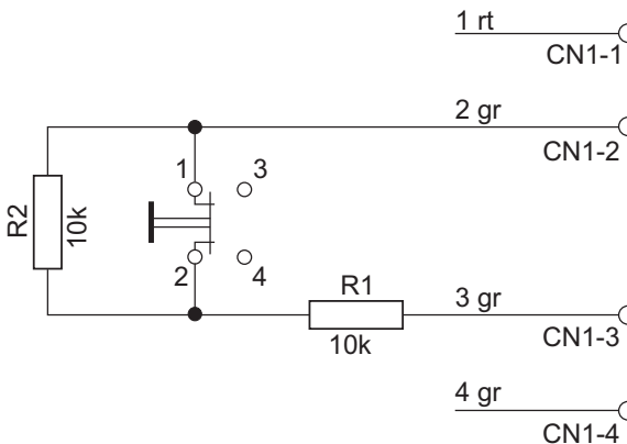
รูป 2.1: การเชื่อมต่อสวิตช์กุญแจเป็นหน้าสัมผัสปิดแบบปกติ (NCC) สำหรับฟังก์ชันกุญแจล๊อค
