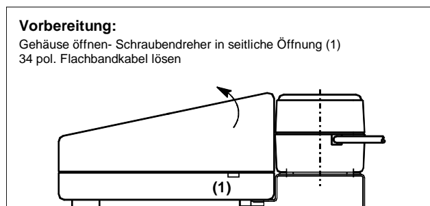
Abb. 7 Gehäuse öffnen
