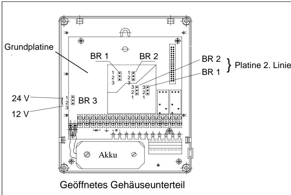
Abb. 1 24/ 12 V- Umschaltung
