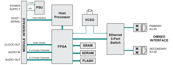
Devre şeması
