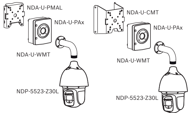
Рис. 2: Мачтовый кронштейн (IP66); угловой кронштейн (IP66)
