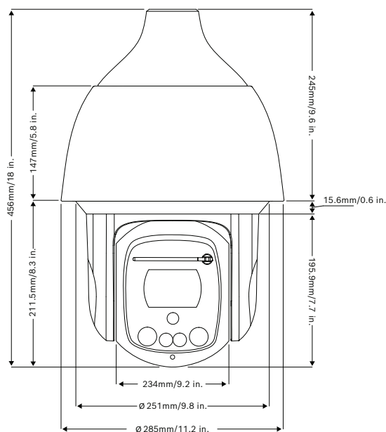
寸法図
