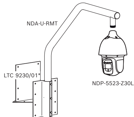
図. 3: ルーフ マウント (IP66)
