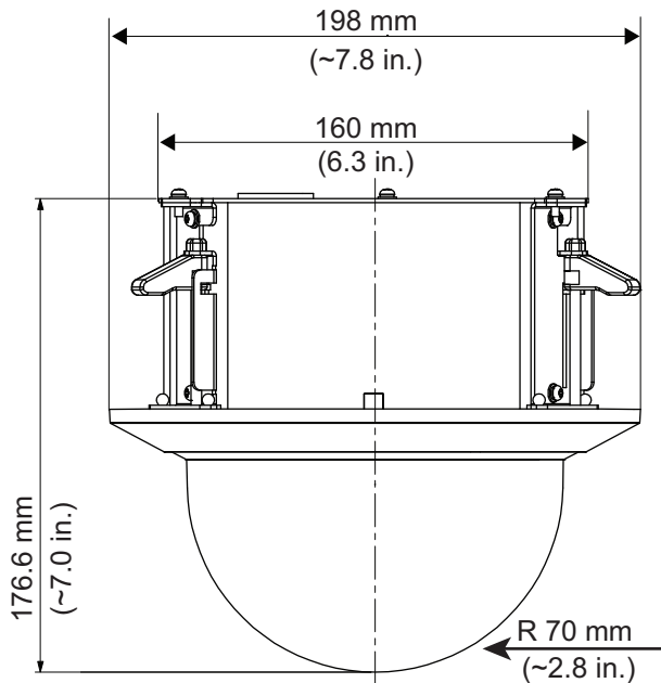
Rys. 1: Model sufitowy
