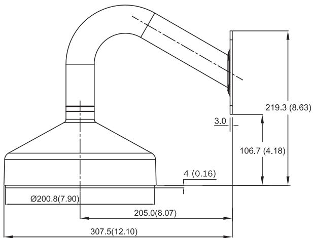
VDA-832FHD-WMT dimensioni installazione a parete
