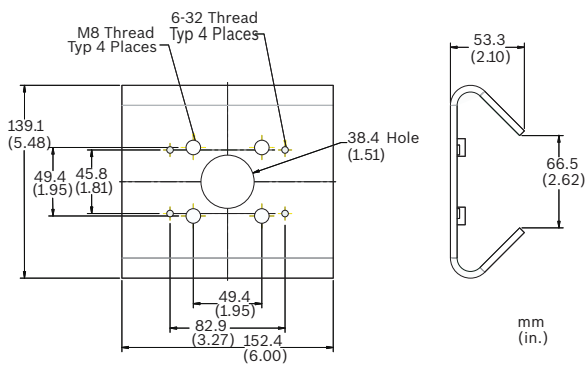
LTC 9213/00 dimensioni adattatore per installazione su palo
