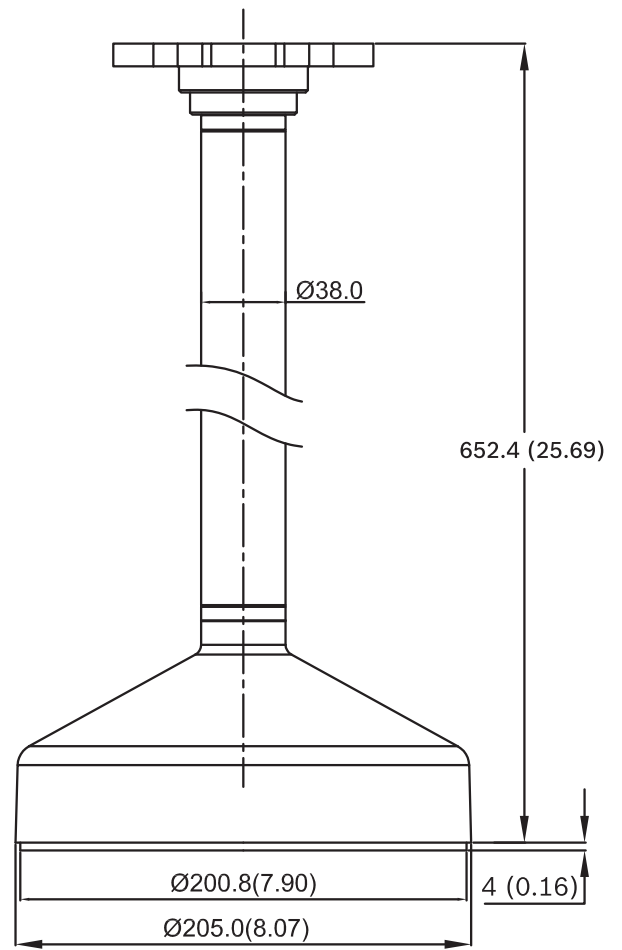
VDA-832FHD-PMT dimensioni installazione su tubo
