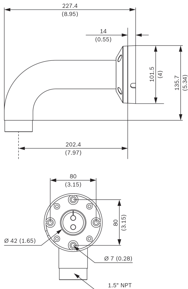
Подвесной настенный кронштейн NDA-U-WMT Размеры в мм
