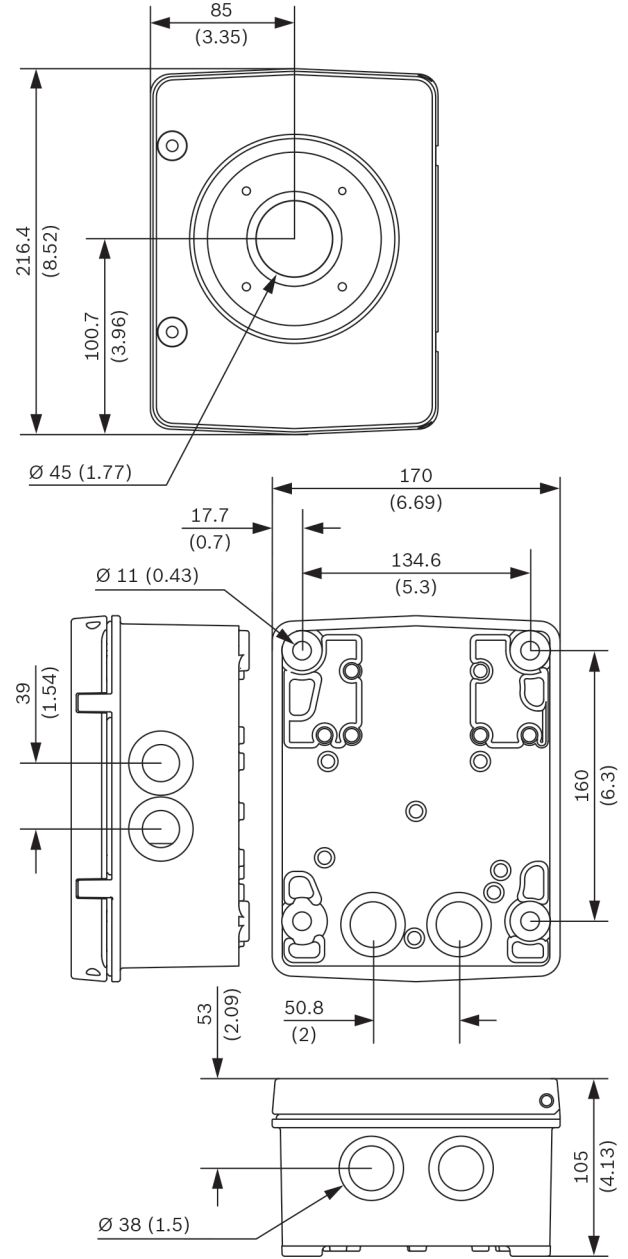
尺寸 (单位: 毫米 (英寸))
