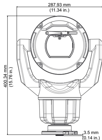
尺寸图
