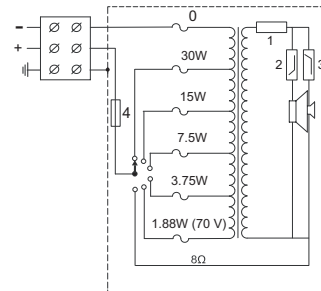
Sơ đồ nối mạch (1: Bộ giới hạn Thu động, 2: Bộ Lọc Tần Số Thấp, 3: Bộ Lọc Tần Số Cao, 4: Cầu chì nhiệt)
