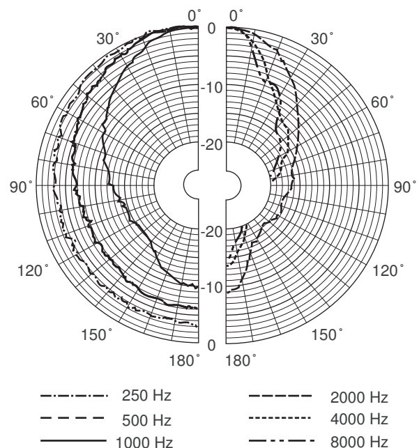
Diagrama polar (medido en ruido rosa)
