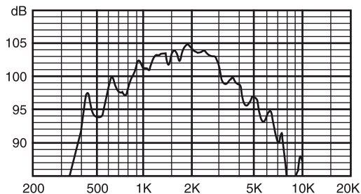
Resposta de frequência
