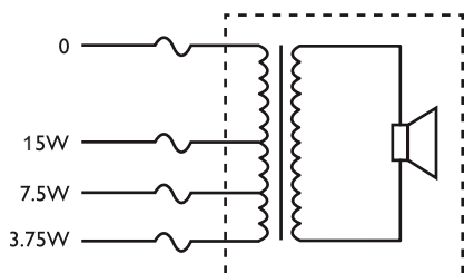
Esquema do circuito
