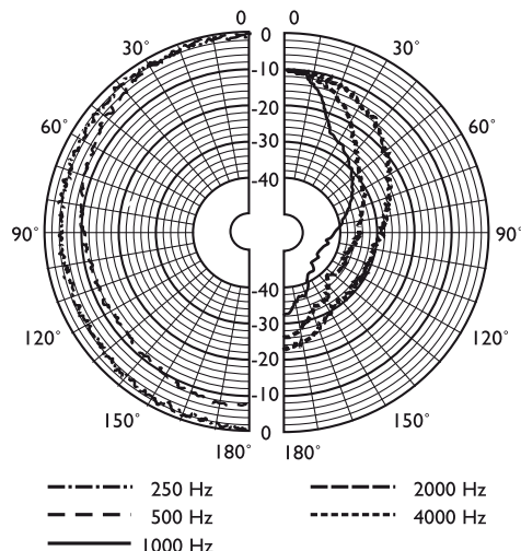
Diagrama polar (medido com o ruído rosa)
