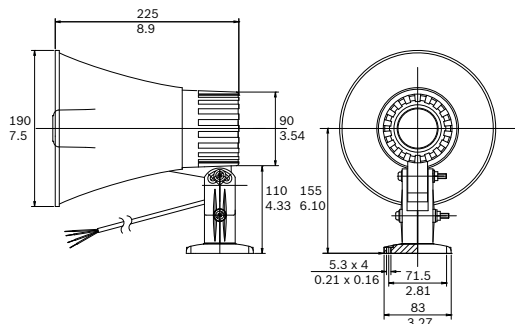
Dimensões em mm (pol.)
