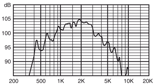
Frekvenciaátvitel
