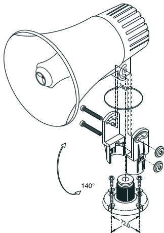
Telepítés
