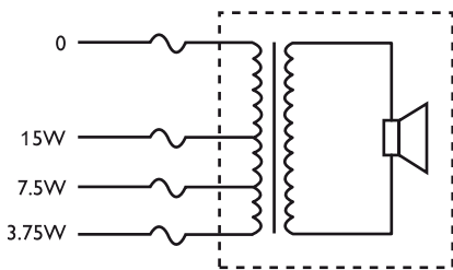
Kapcsolási rajz
