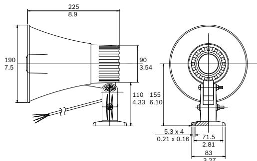
Rozměry v mm (palcích)
