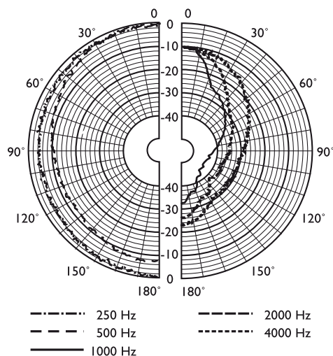
Polární diagram (měřeno s růžovým šumem)
