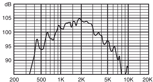
Kmitočtová charakteristika
