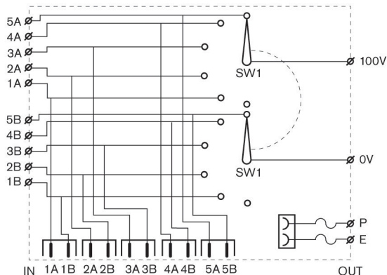
Esquema do circuito LBC 1430/10
