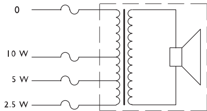
Sơ đồ nối mạch
