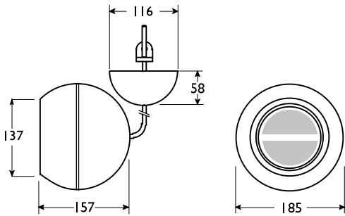
Kích thước (tính theo mm)
