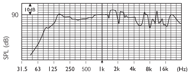
Hồi đáp tần số
