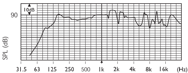
Απόκριση συχνότητας
