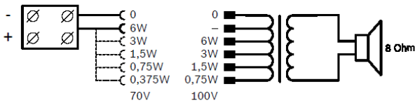
Diagrama de circuitos
