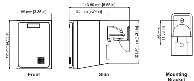
Loa vệ tinh gắn bề mặt và giá đỡ
