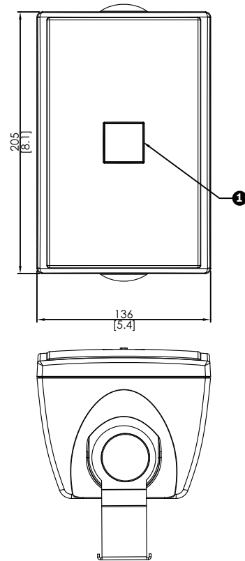
Πρόσωση και κάτοψη σε mm (in.). (1) Περιστρεφόμενο λογότυπο
