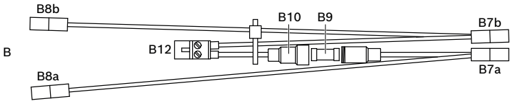
Afbeelding 4.2: Voeding (accu)
