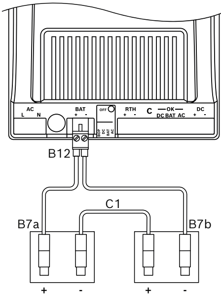
Afbeelding 3.4: 24 V-modus
