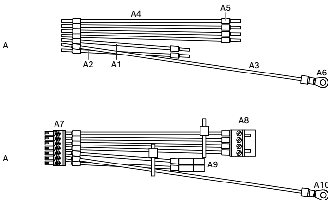
Afbeelding 4.1: Voedingskabel (AMC2)
