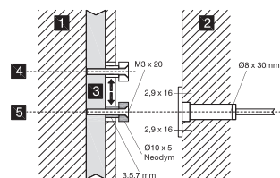
Fig.1 Disposition de montage frontale
