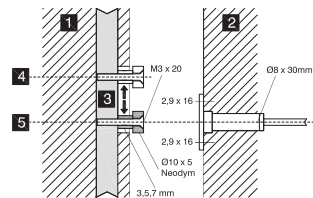
Mindestabstand Fenster – Rahmen 12mm
