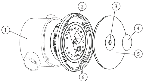
Fig. 1: Descripción general del sistema
