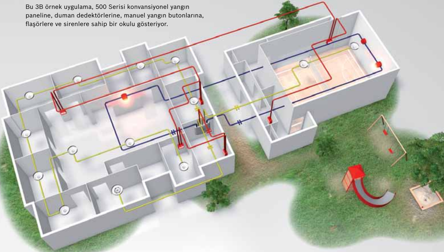
Konvansiyonel Yangın Paneli 500 serisi
