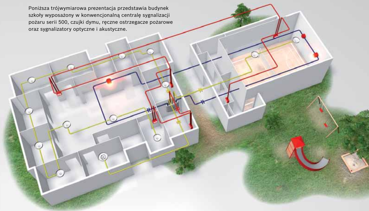
Konwencjonalna centrala sygnalizacji pożaru serii 500
