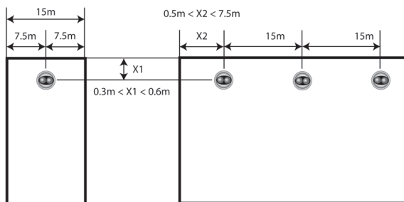
Rys. 2: Montaż (płaski strop)
