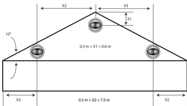
Rys. 4: Montaż (dach dwuspadowy)
