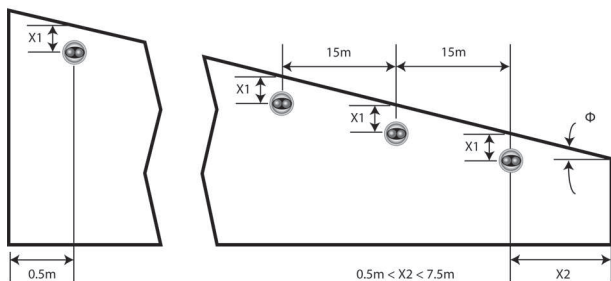
Rys. 3: Montaż (dach spadzisty)
