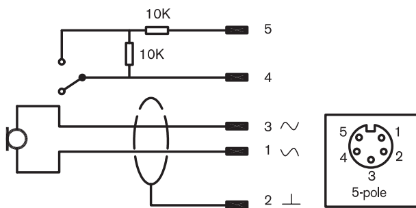
Sơ đồ nối mạch
