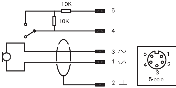
Devre şeması
