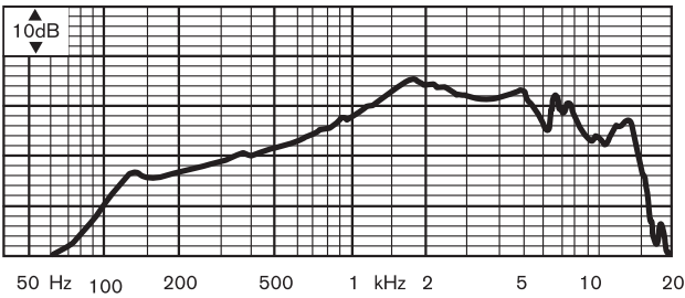
Frekans yanıtı
