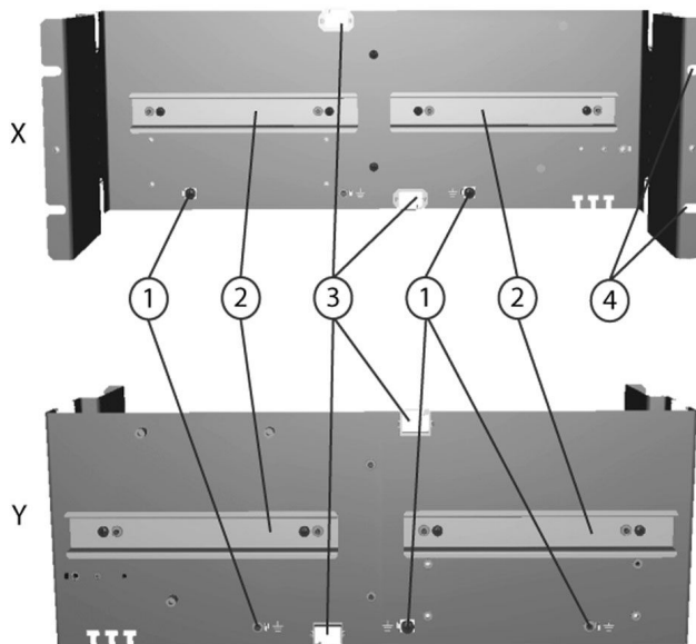
Вид спереди и сзади шасси АЕС-РАNЕL19-4DR:
