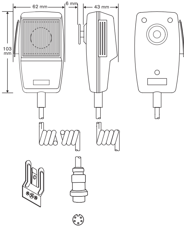
Mitat millimetreinä
