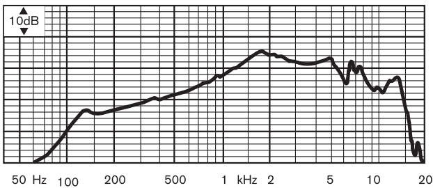
Taajuusvaste
