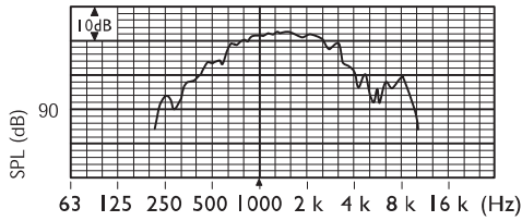
Απόκριση συχνότητας
