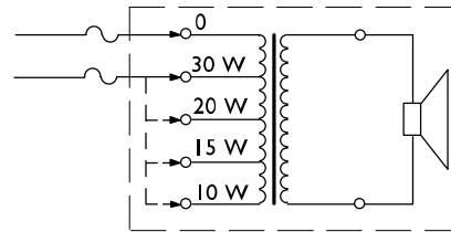
Διάγραμμα κυκλώματος
