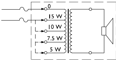
Διάγραμμα κυκλώματος
