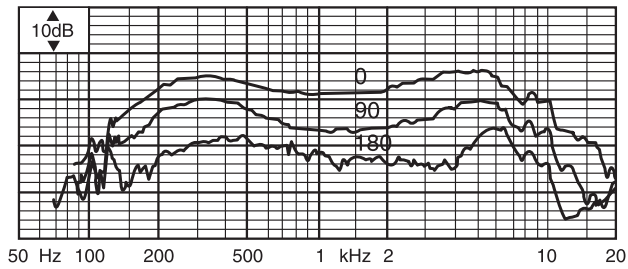
Απόκριση συχνότητας
