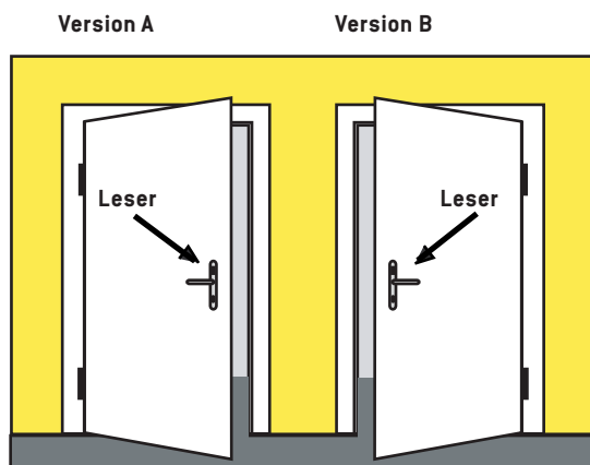
Tür DIN links Öffnung rechts einwärts
