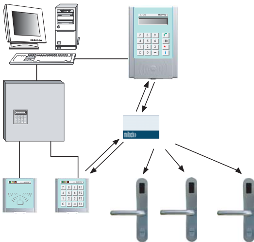
Abb. Kombination von Zutrittskontrolle und Offline-Türterminals.
