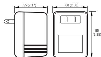
EXPS.004 Gehäuse
