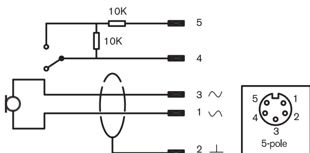
Schéma zapojení
