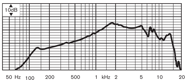
Kmitočtová charakteristika
