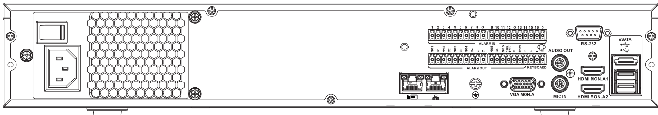
图片 1: DIVAR 5000网络后面板 (无PoE)
