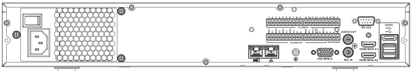
Fig. 1: Panneau arrière DIVAR 5000 network (non PoE)
